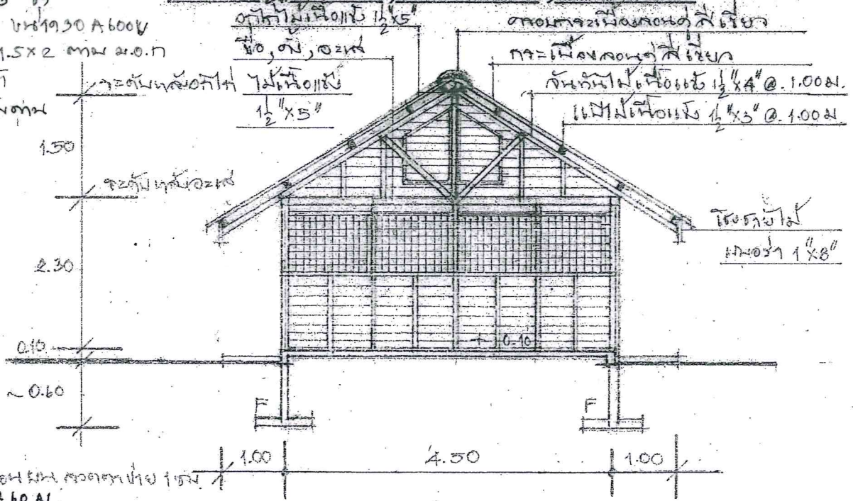
รูปตัด 1-1 1:75 4-Ø12 มม. 17-Ø6 มม. @ 0.15 Ø 6 มม. @ 0.20 มม.
